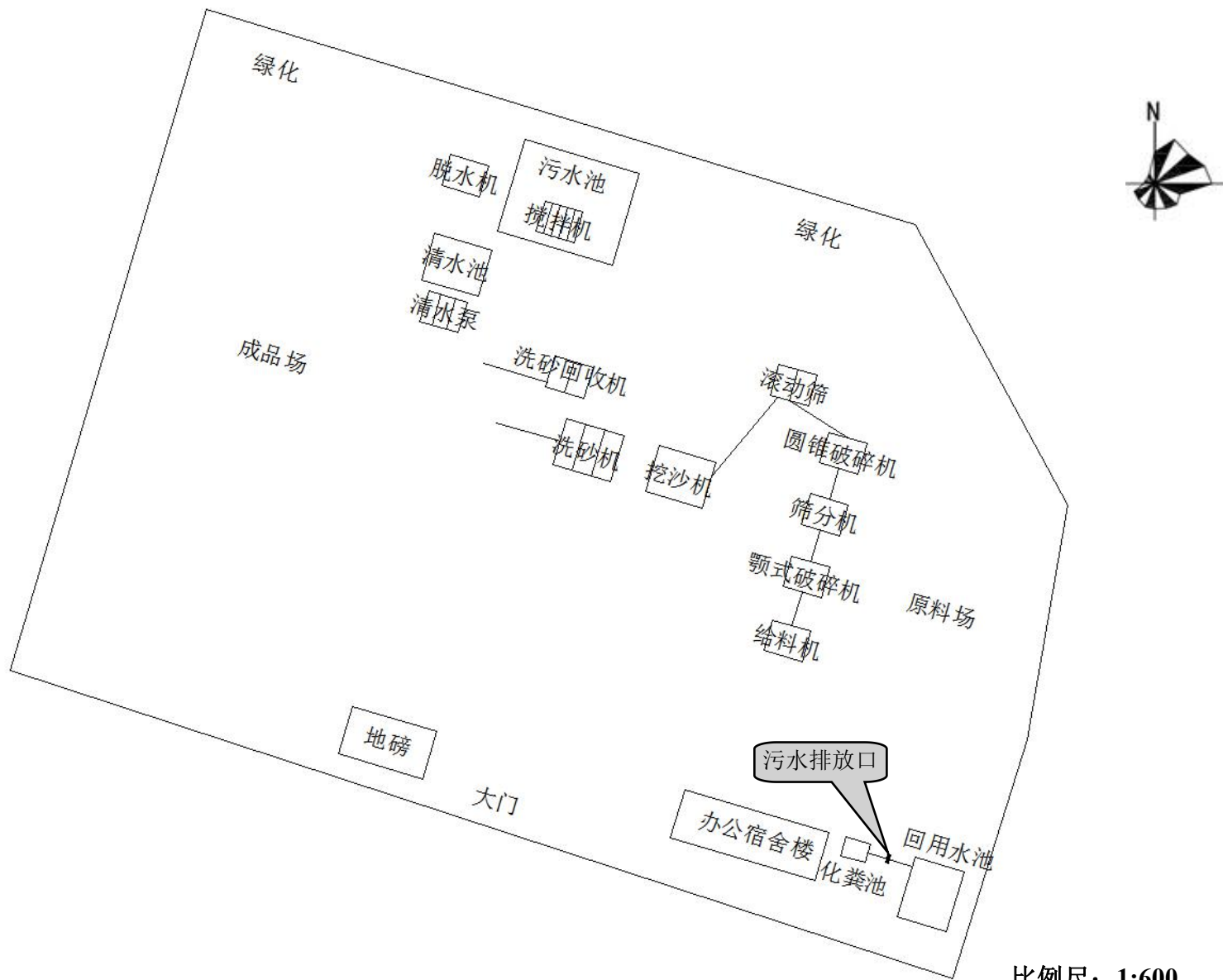
附图八：项目平面布置图
