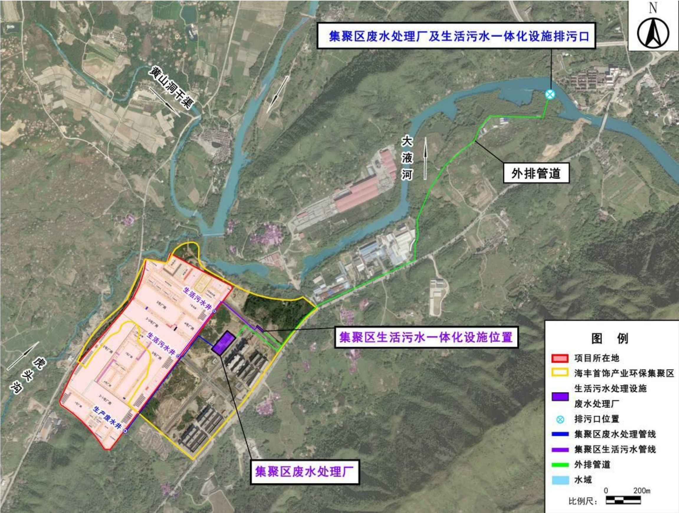
附图 19a 本项目废水接入海丰首饰产业环保集聚区污水处理厂及生活污水一体化设施管线图
