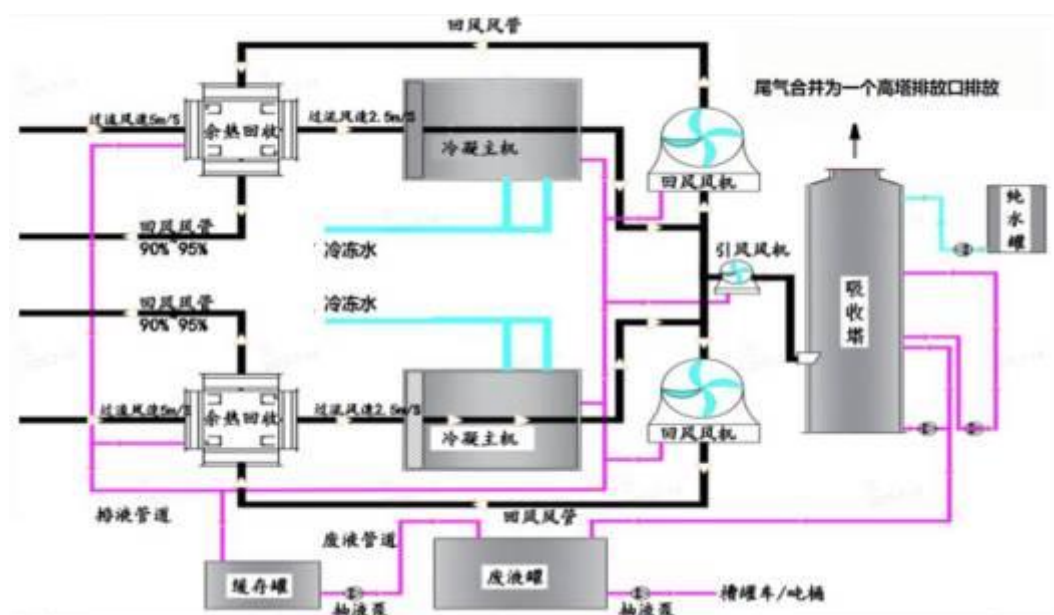
图 4-2 涂布废气处理流程图
