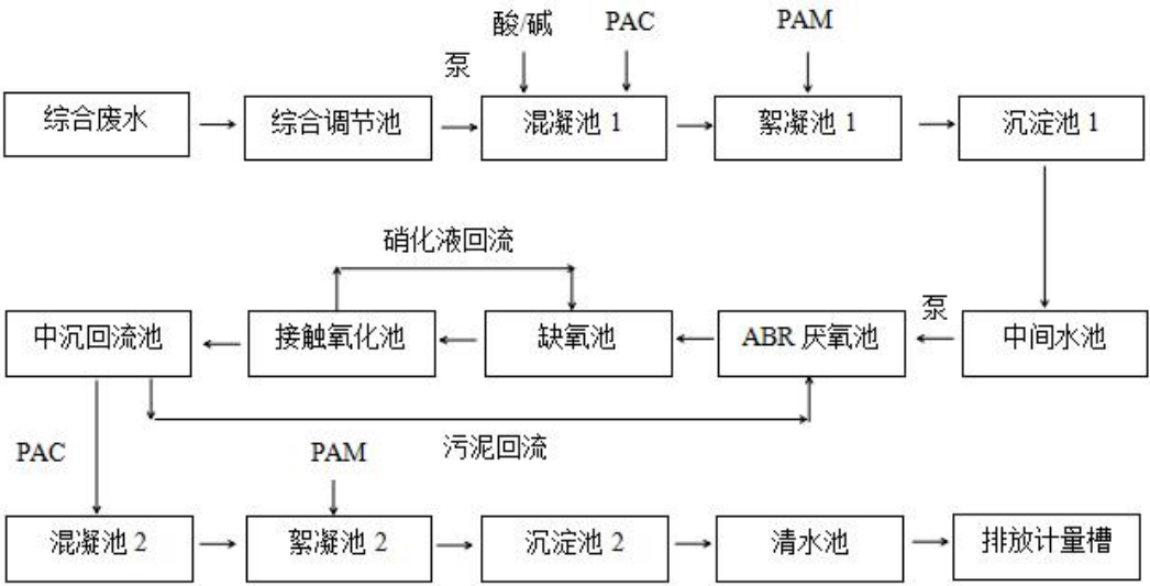
图 4-5 综合废水处理系统工艺流程图
