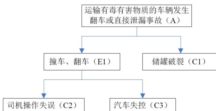
图 1.7-1 事故树
