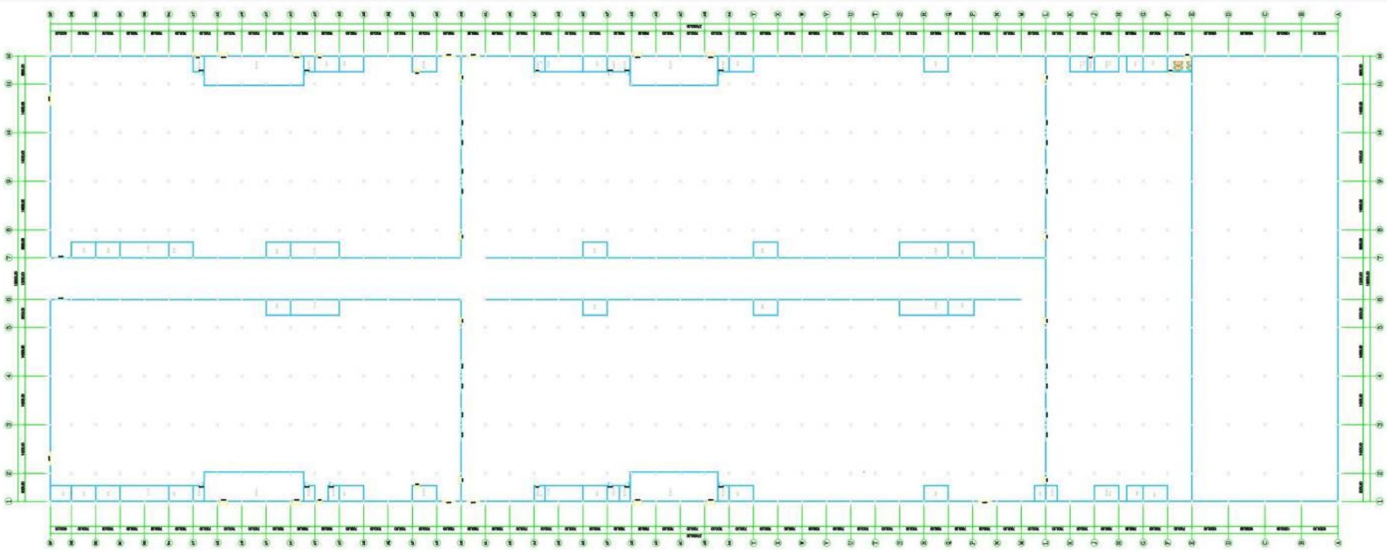
海丰5#-1F厂房平面布局方案图
