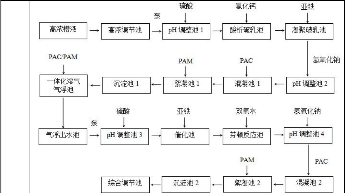
图 4-4 高浓度废水预处理系统工艺流程图
