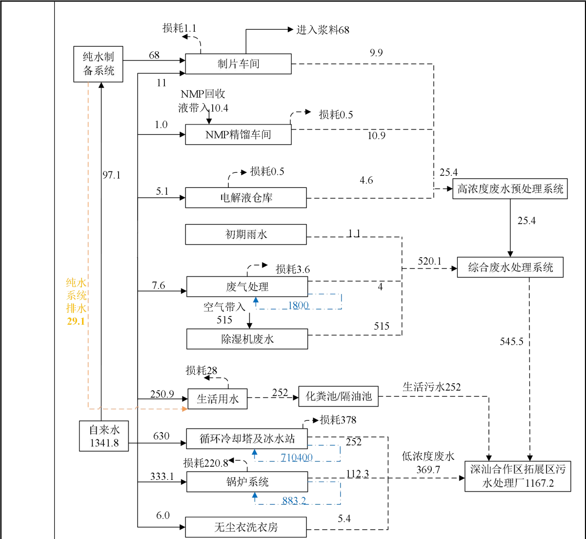
图 2-3 本项目水平衡图 (m³/d)
